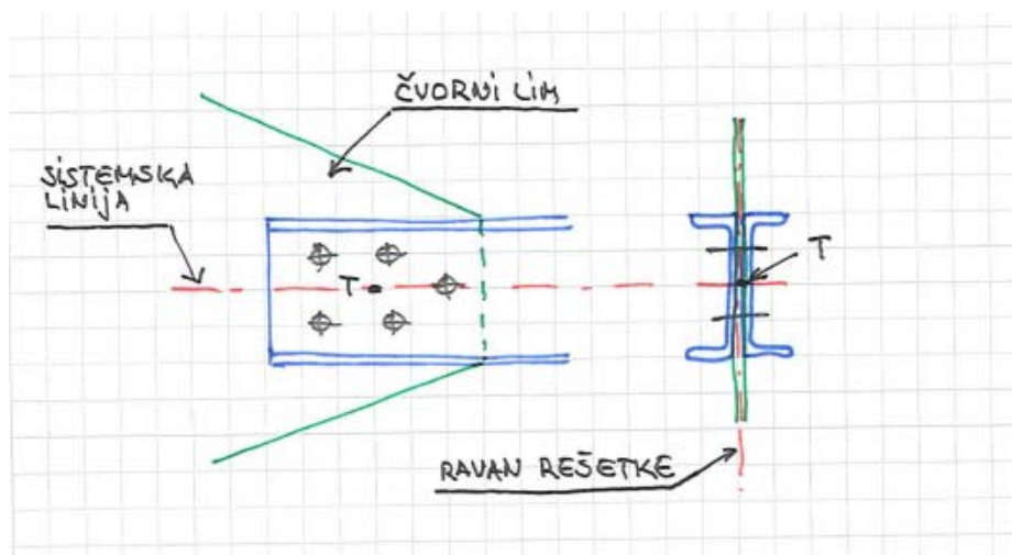
Centrisani i štap i veza na sistemsku liniju i u ravni rešetke i van ravni rešetke.
